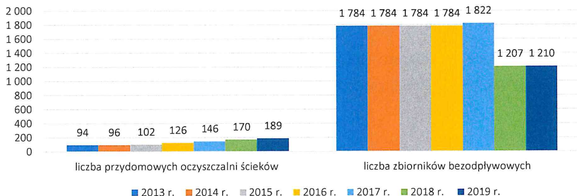
WYKRES 3. Liczba przydomowych oczyszczalni ścieków oraz liczba zbiorników bezodpływowych [szt.] w latach 2013–2019
